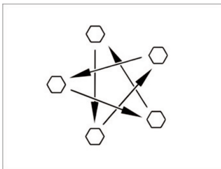
Fig. 168: Serrare in sequenza incrociata i dadi o i bulloni di fissaggio ruota
