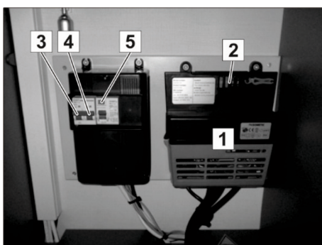
Fig. 67: Convertitore (alimentatore di rete) (1) e interruttori automatici
