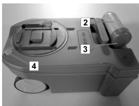
Fig. 158: Svuotare il serbatoio acque nere
