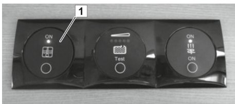
Fig. 98: Interruttore ON/OFF per la preparazione di acqua calda sanitaria
