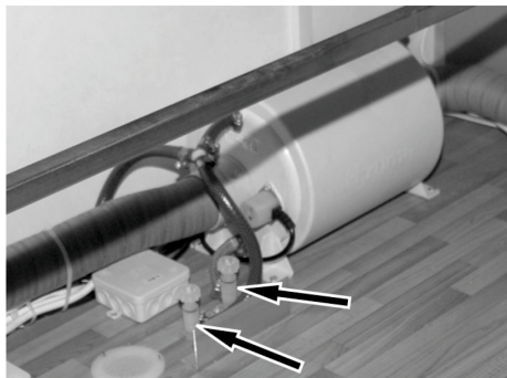
Fig. 135: Valvole di scarico
