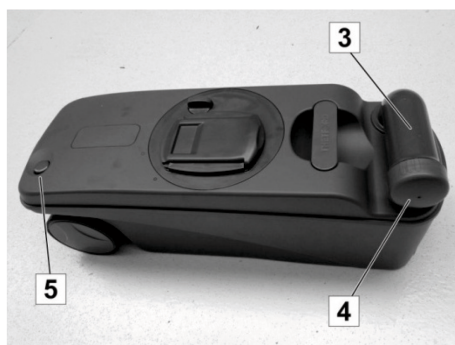
Fig. 155: Svuotare il serbatoio acque nere
