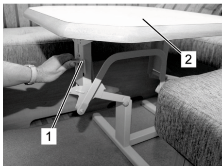
Fig. 138: Tavolo con telaio di sollevamento
