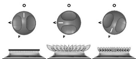
Fig. 161: Posizione degli elementi di comando: OFF, Fiamma alta, Fiamma bassa
