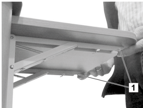
Fig. 145: Allentare il bloccaggio
