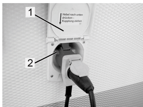
Fig. 99: Allacciamento alla rete
