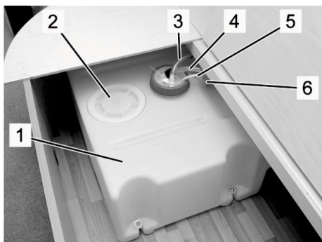
Fig. 92: Serbatoio dell'acqua fresca, esempio
