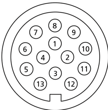
Fig. 2: Spina a 13 poli
